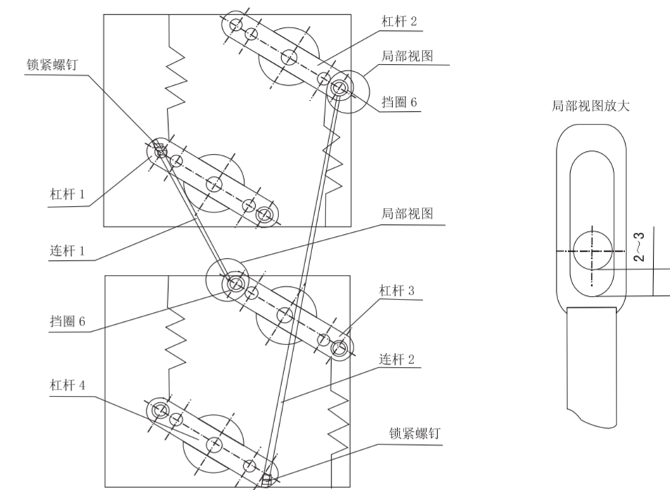
两台断路器之间的硬杆锁连接示意图。
