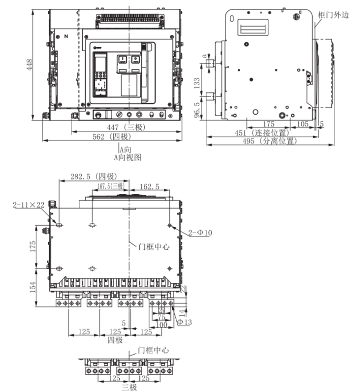
19.8 TGW1N-4000(In=2500-3200A)抽屉式断路器外形尺寸与安装尺寸图
