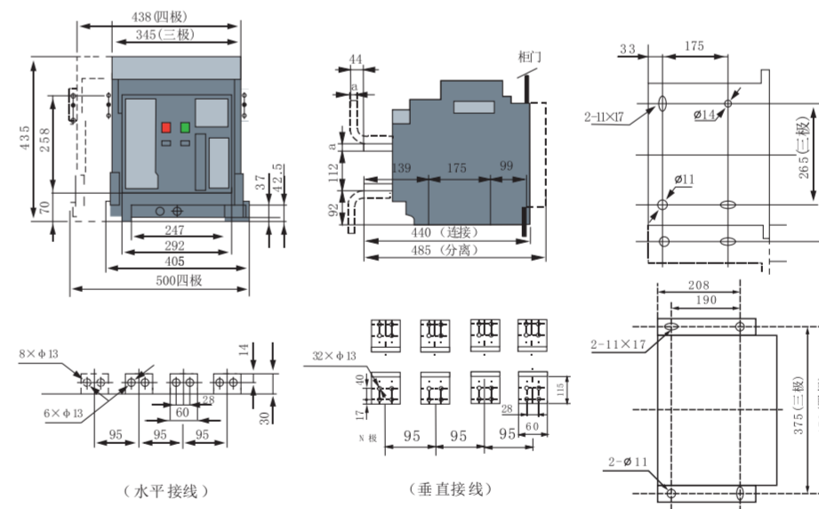
19.2 TGW1N-2000/TGW1N-2000H抽屉式断路器外形尺寸与安装尺寸图。
