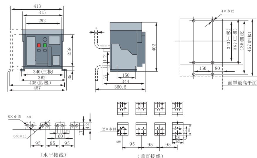
19.1 TGW1N-2000/TGW1N-2000H固定式断路器外形尺寸与安装尺寸图。
