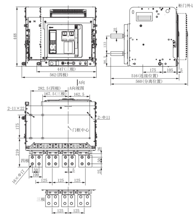
19.10 TGW1N-4000(In=3600-4000A)抽屉式断路器外形尺寸与安装尺寸图。
