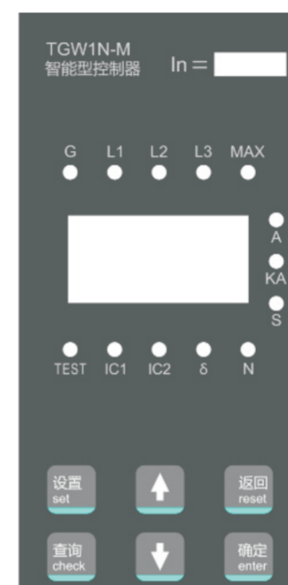
20 控制器面板指示图及操作
